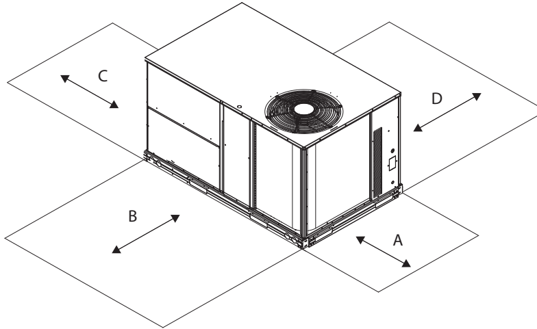
Fig. 2 - Dimensions RGS036-072
