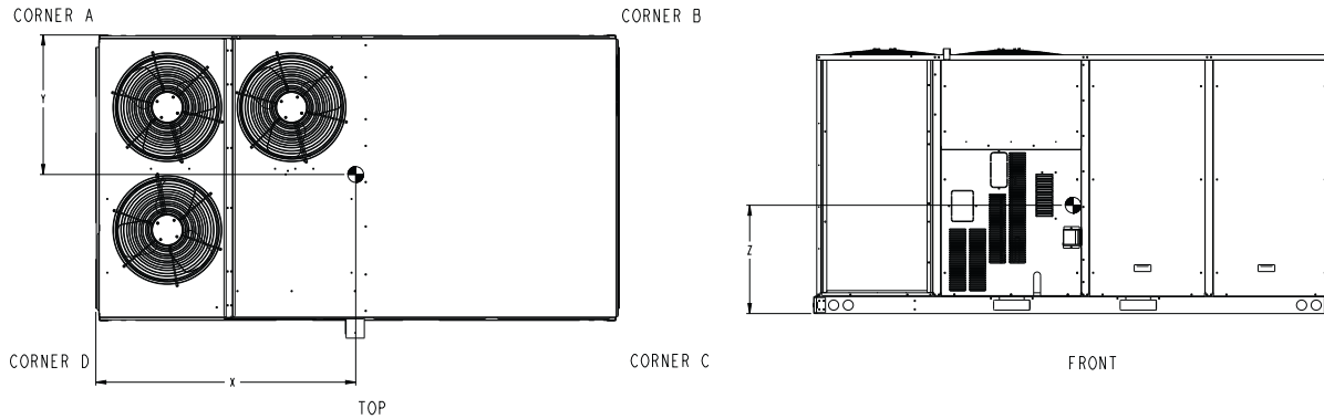
Fig. 13 - Dimensions RGS180
