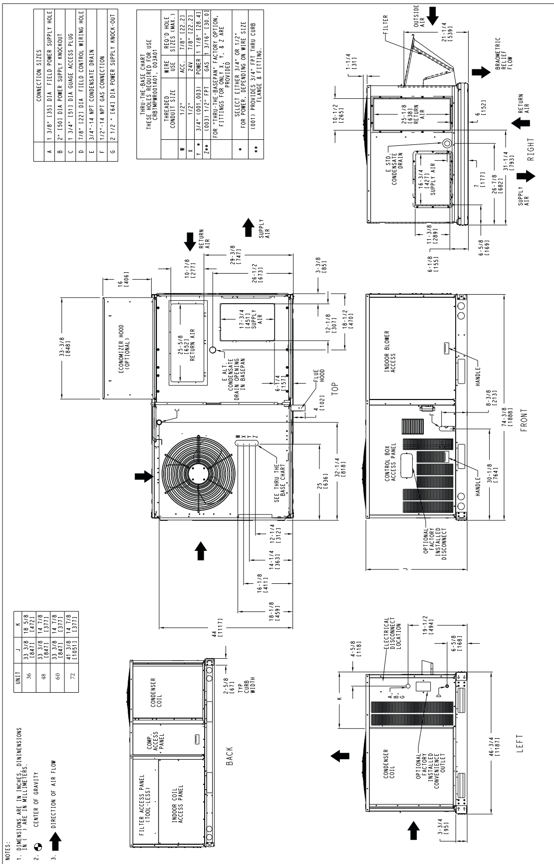
Fig. 1 - Dimensions RGS036-72
