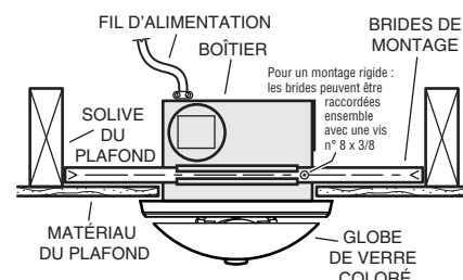
SOLIVES ESPACÉES DE 60,9 CM (24 PO) CENTRE À CENTRE
